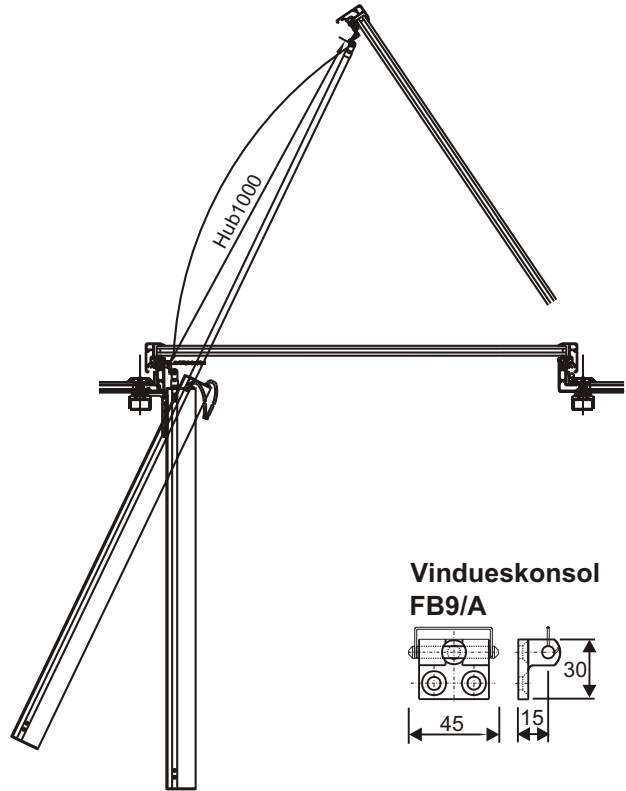
Skydeklap-konsol K26/B/XL
