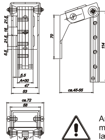
Skydeklap-konsol K27/B/XL for motorhusets underste føringsspor
